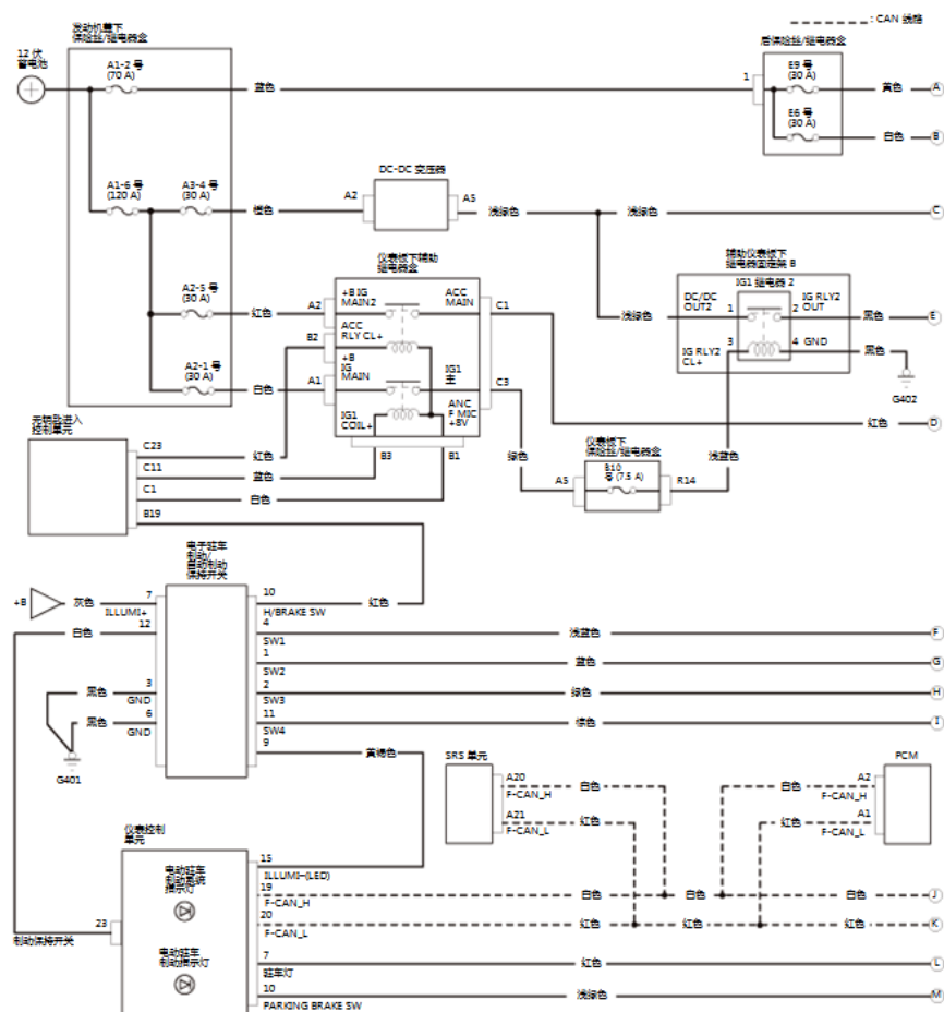
电子驻车制动系统电路图
